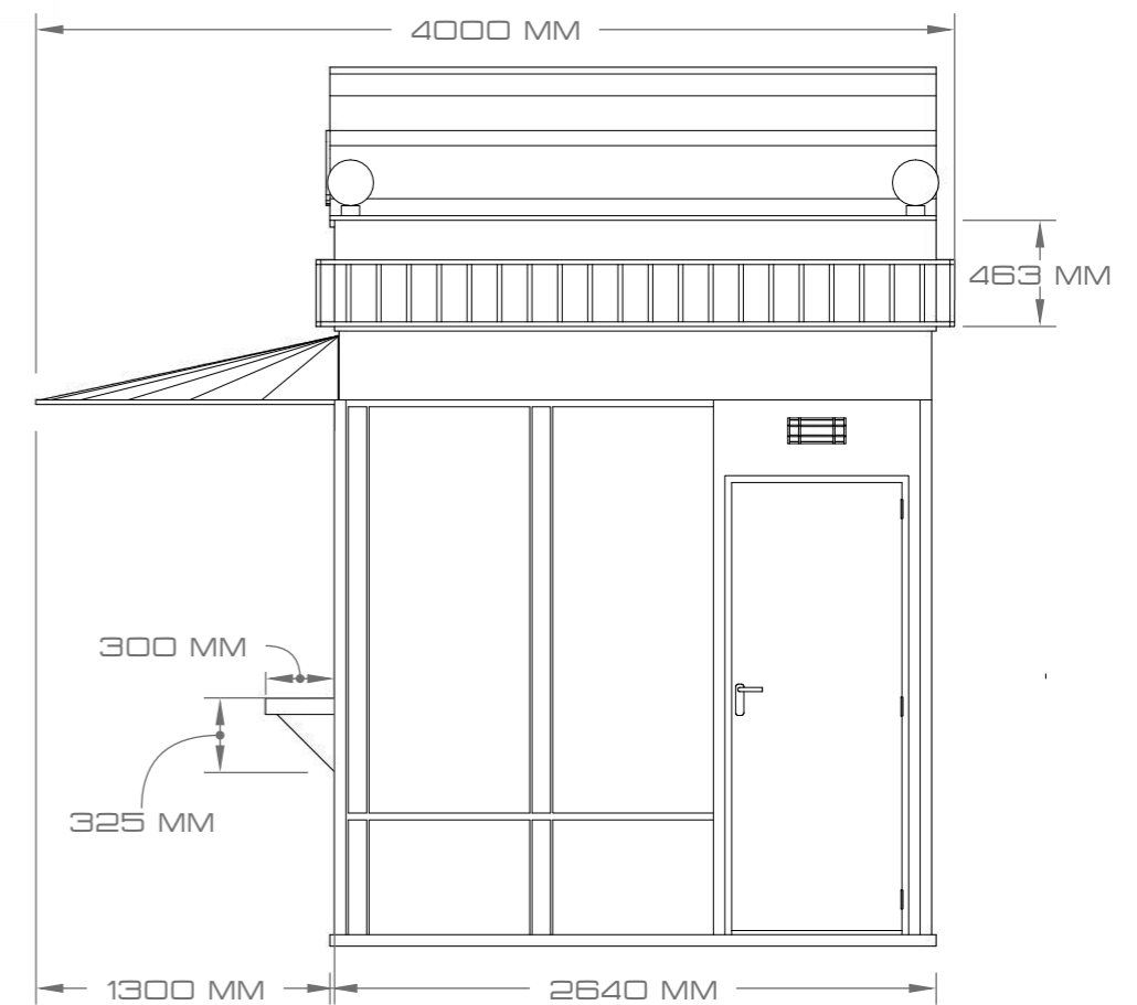
KIOSK RIGHT SIDE
