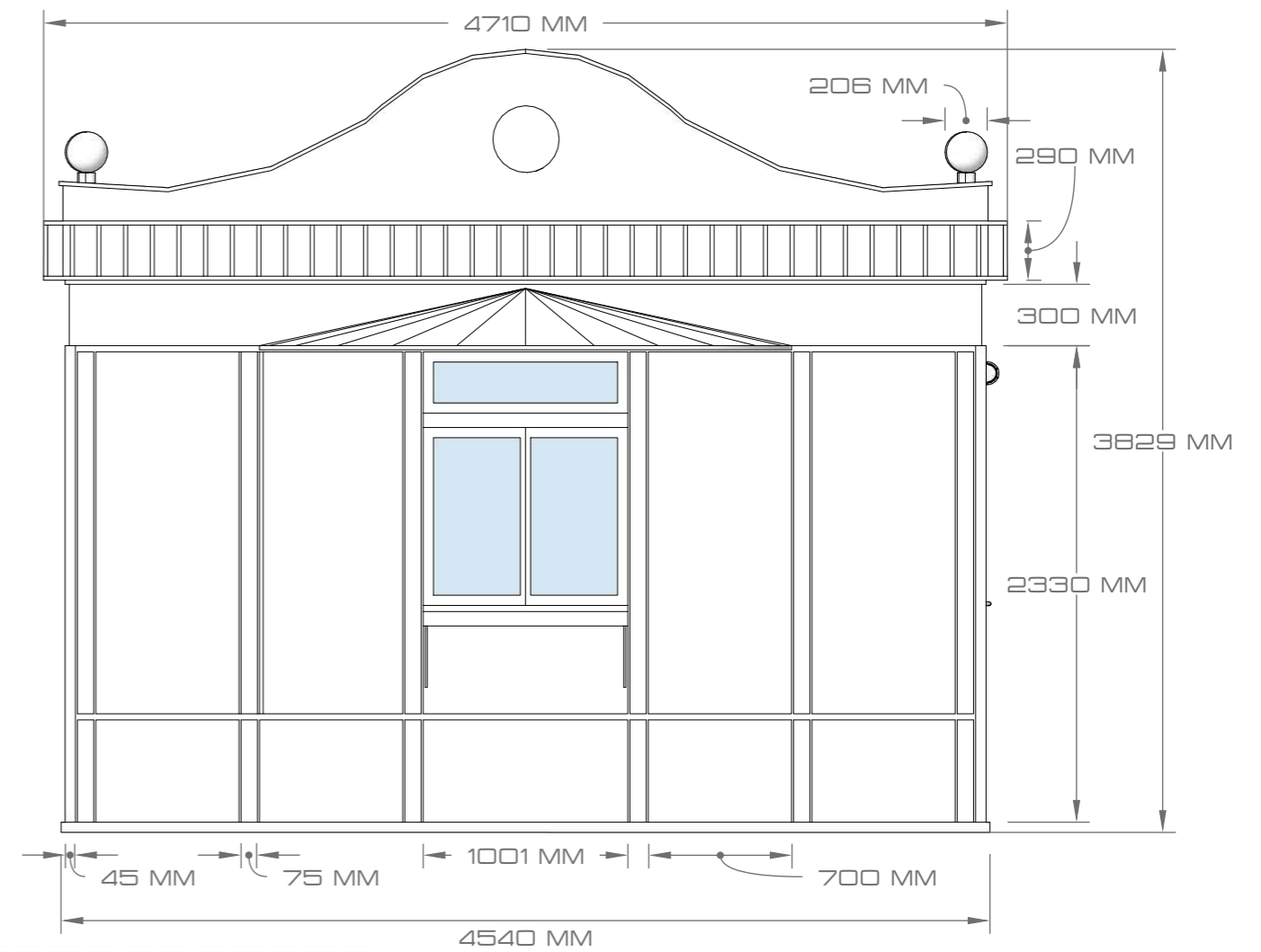
KIOSK FRONT
